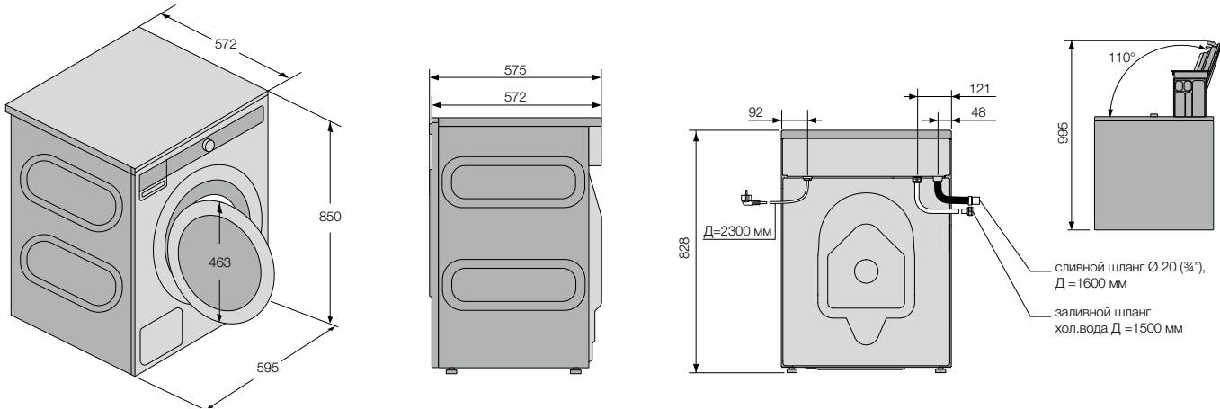
Схема установки
