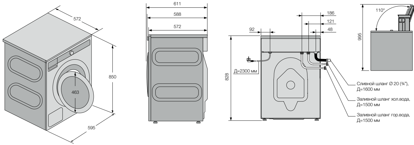
Схема установки
