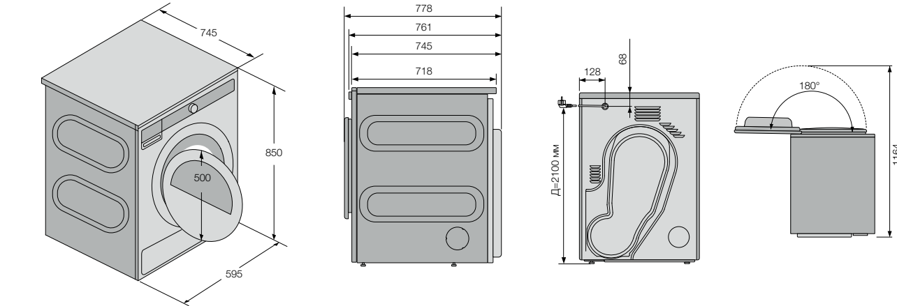
Схема установки
