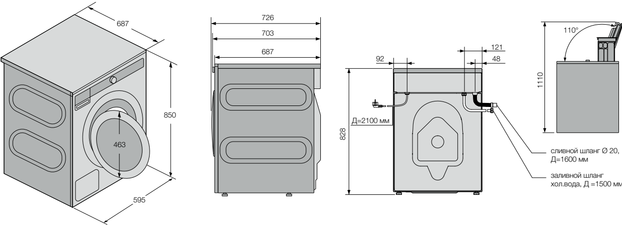
Схема установки
