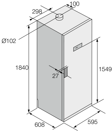
Схема установки
