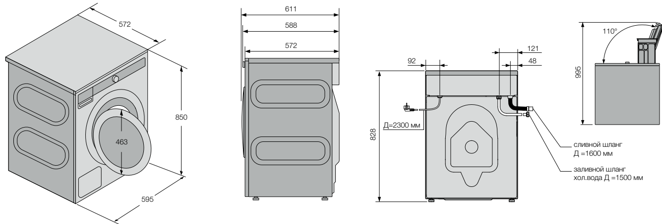
Схема установки
