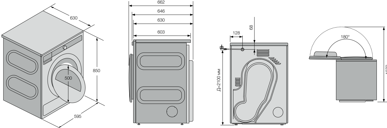
Схема установки
